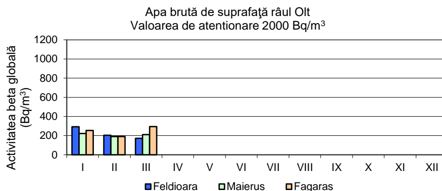
Fig. 20. Activitatea beta globală la 5 zile pentru apa de suprafață Râul Olt
