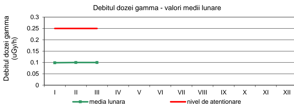
Figura 16. Debitul dozei gamma
