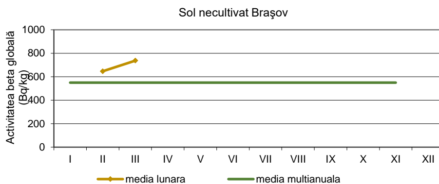
Fig. 21. Activitatea beta globală la 5 zile pentru sol necultivat
